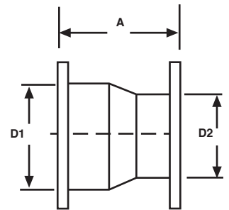
FLANGE / FLANGE
