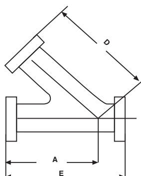
FLANGE / FLANGE
